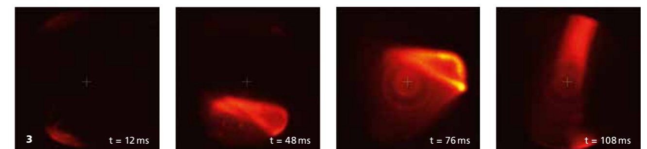
3 Der LITRAN-Bildkonverter als schnelle Kamera: Infrarotaufnahmen (bei ca. 3 \mu\text{m} ) der Ausbildung einer (Feuerzeug-) Gasflamme. Neben der Kontur der Flamme ist das thermische Leuchten des heißen Wasserdampfes in der Umgebung der Flamme zu sehen. Dieser emittiert Infrarotstrahlung bei einzelnen Wellenlängen, die im Bild als Ringmuster erkennbar sind.
