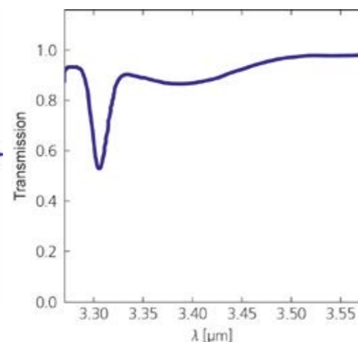
2 Der LITRAN-Bildkonverter als Spektrometer: Das Licht eines thermischen Strahlers passiert eine mit Methan gefüllte Gaszelle und wird von der LITRAN-Kamera aufgenommen. Das Kamerabild wird in ein Spektrum umgerechnet. Aus dem Ringmuster lassen sich Wellenlänge und Stärke der Methanabsorption bestimmen.
