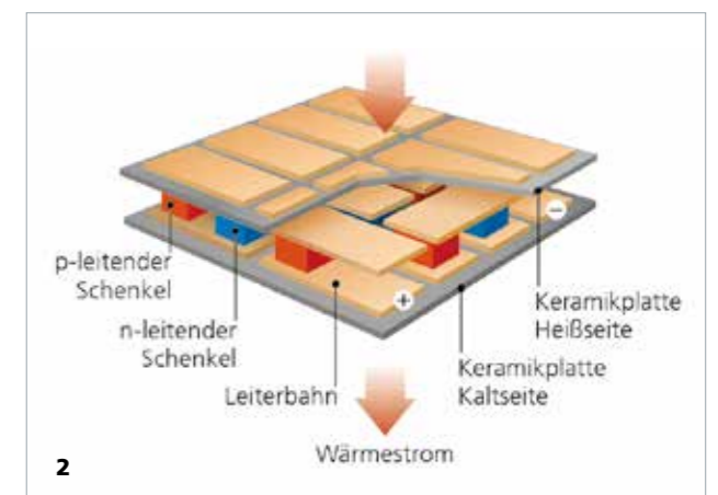
2 Aufbau eines thermoelektrischen Moduls.
